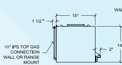
END ELEVATION
